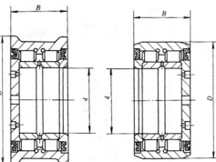
NNUPN3326X3型
