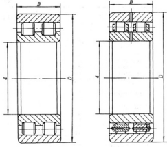
NNUPN3326X3型 (682000型)
