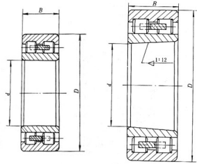
NNUPN3326X3型 (482000型)
