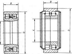
NNUPN3326X3型 (82000型)
