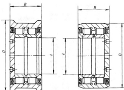
NN000000-2LSV 型 特殊结构的双列圆柱滚子轴承
