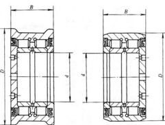
NNFP0000-2LSV 型 NNFP0000-2LSVW 型 特殊结构的双列圆柱滚子轴承
