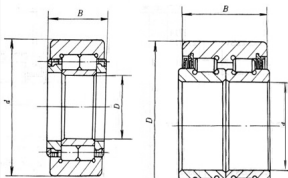
NNJ0000-2Z 型 (462000 型)
