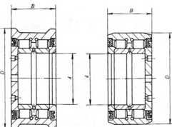
NN0000-2LSV 型
